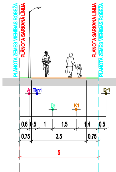
PLĀNOTĀ GĀJĒJU CEĻA ŠĶĒRSPROFILS GRIEZUMS 2 - 2
