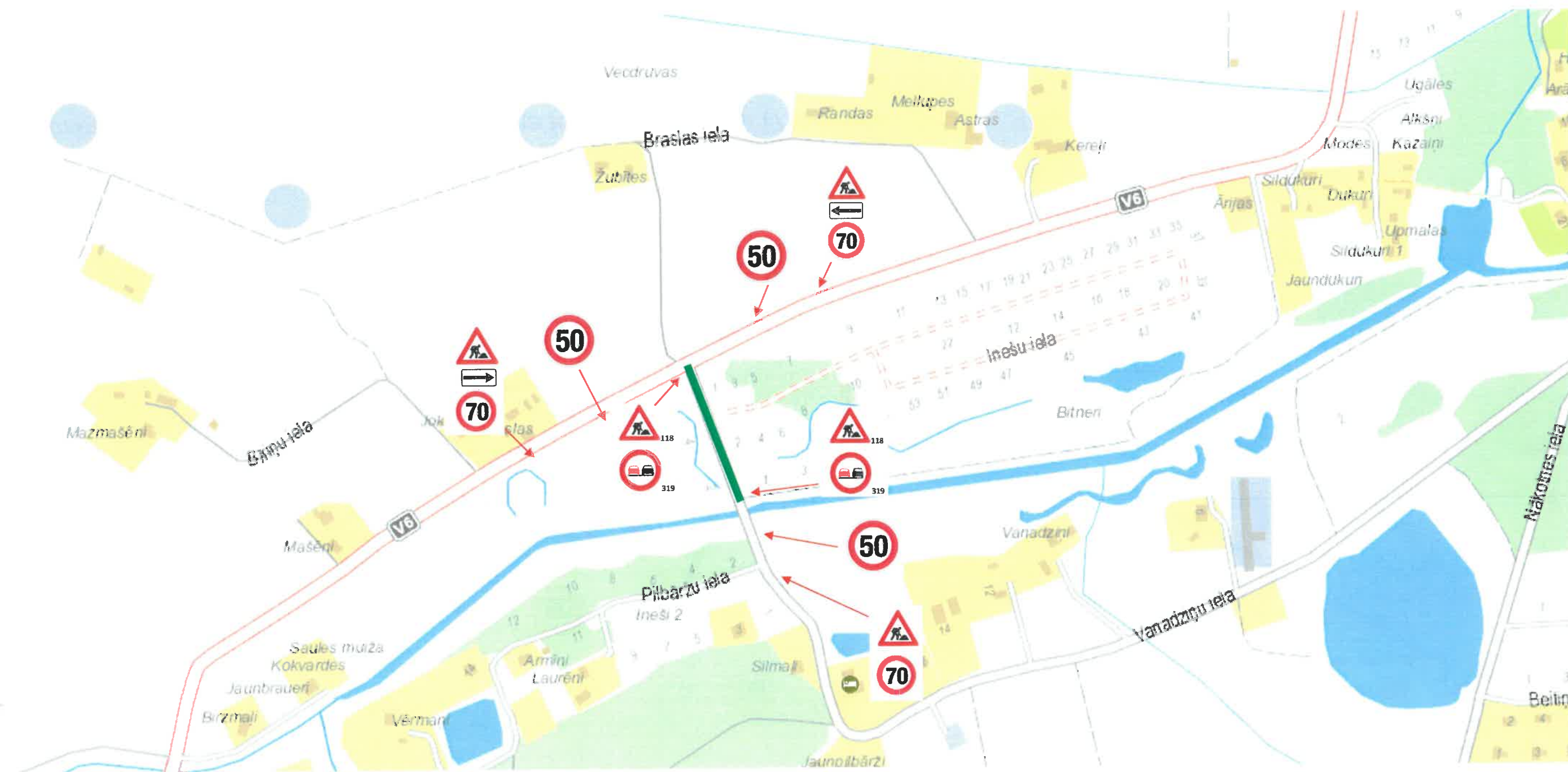
Vanadziņu iela, Ķekava. Satiksmes org. shēma būvdarbu laikā.
