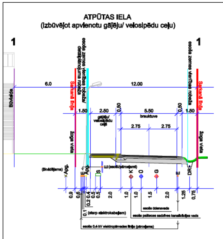
2.att. Atpūtas ielas rekomendējošs šķēršprofils velosipēdiņam.
