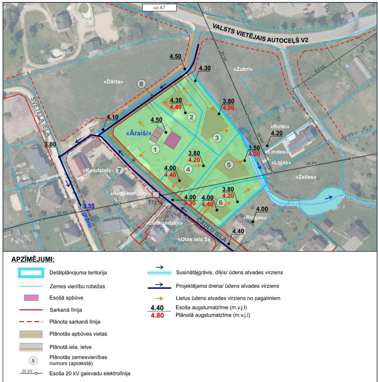
4.5.attēls. Meliorācijas sistēmas priekšlikums 13
