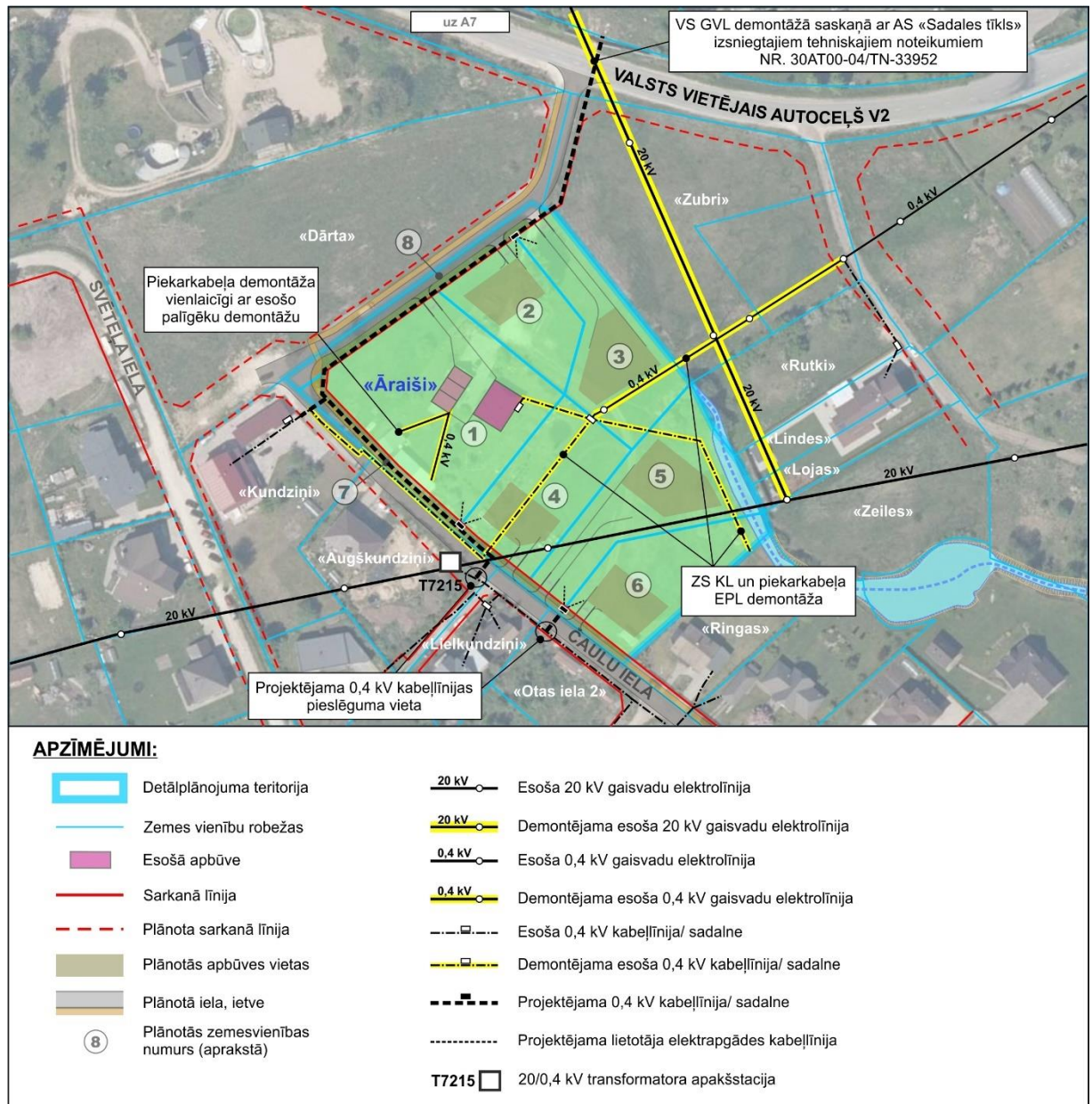
4.7.attēls. Elektroapgādes risinājumu priekšlikums 17
