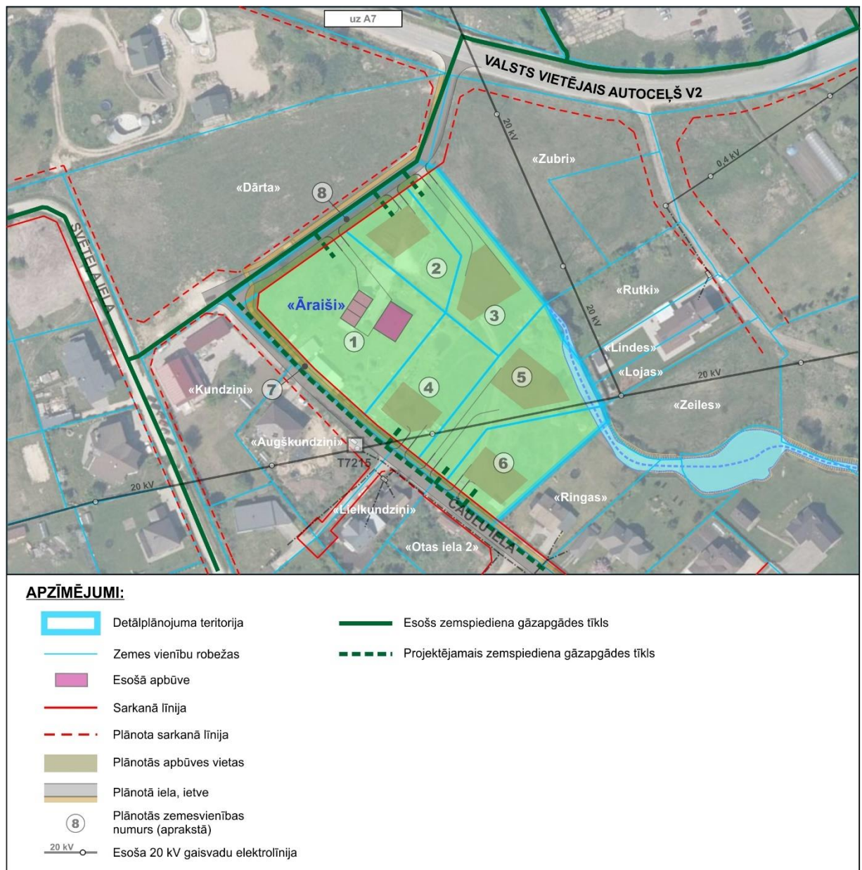
4.8.attēls. Gāzapgādes risinājumu priekšlikums 18
