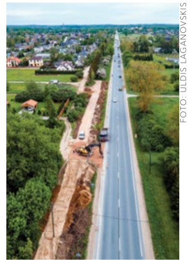
Velocēļa gar autoceļu A7 pirmā posma izbūve Ķekavā.
