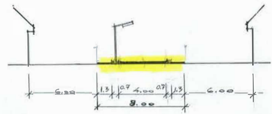
CEĻAS ŠĶĒRSPROFĪLS M 1:200
